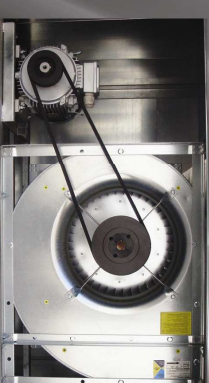
Ventilador centrífugo de doble aspiración, transmisión por correas y poleas (Extractor). Double inlet centrifugal fan with belts and pulleys (Generator).
